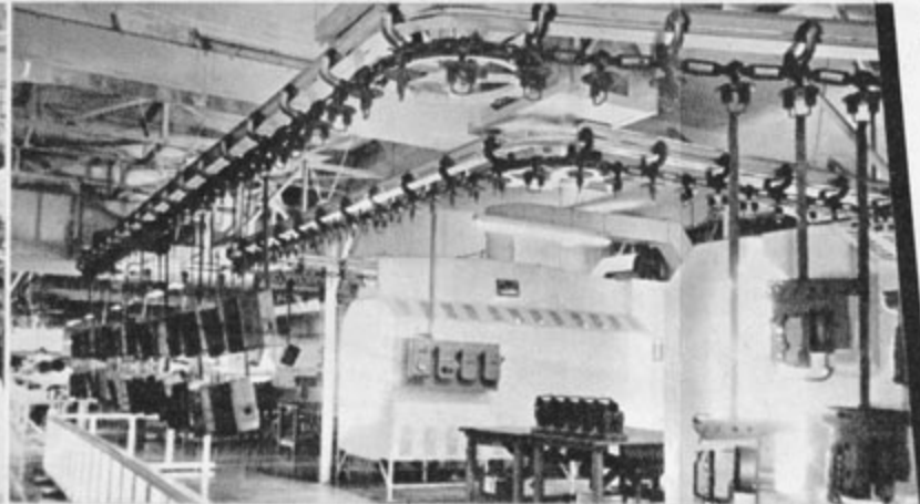
赤外線乾燥炉の並ぶ、オートメーション化された塗装工場
